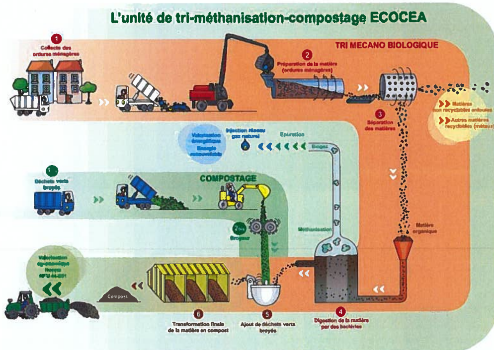
Figure 6 : Schéma de fonctionnement d'ECOCEA
