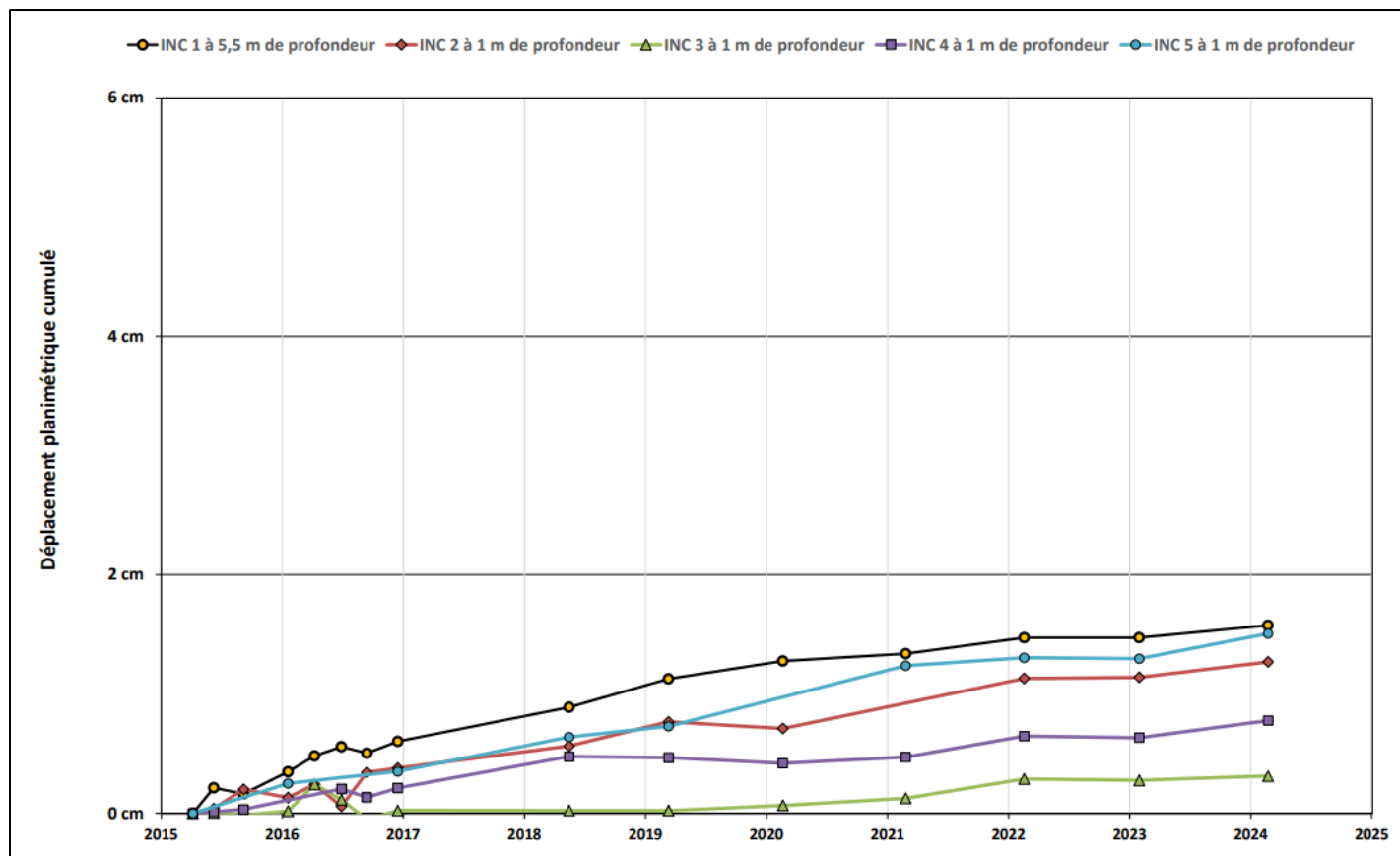
Figure : déplacement horizontal à 1m de profondeur (inclinométrie) Évolution depuis 2015
