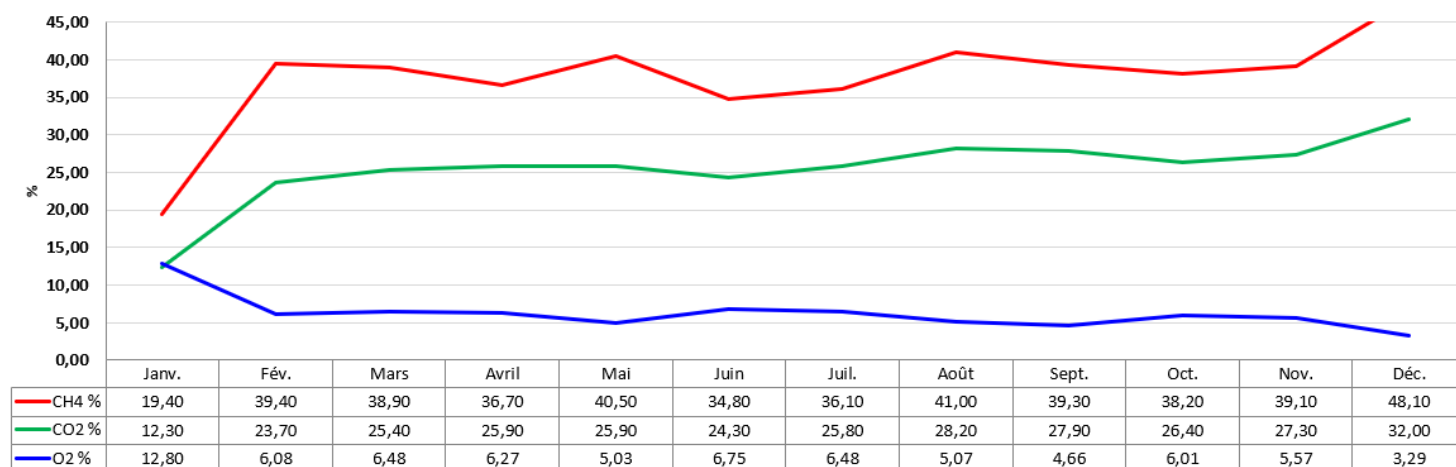
Composition 2023 du biogaz - Suivi SMET
